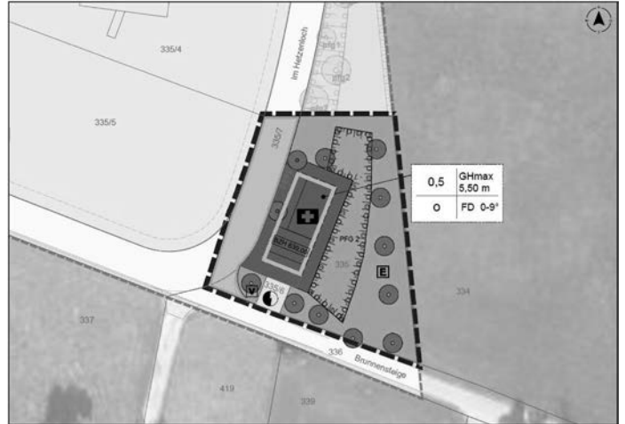
Auszug aus dem Lageplan des Bebauungsplans „Gewerbegebiet Hetzenloch, 1. Änderung“ in Böhmenkirch-Schnittlingen
